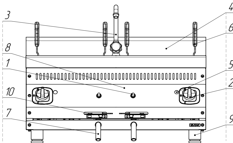
Рис. 2. Газоварка ГВК-80/2Н
